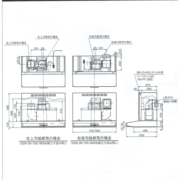
SSR-3R、別売品SSRV取付寸法図
